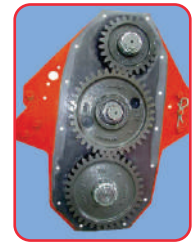
Transmisión lateral de engranes
